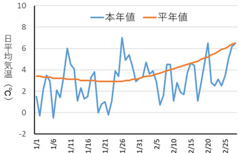
図 令和4年1～2月の日平均気温の推移 (甲府)
