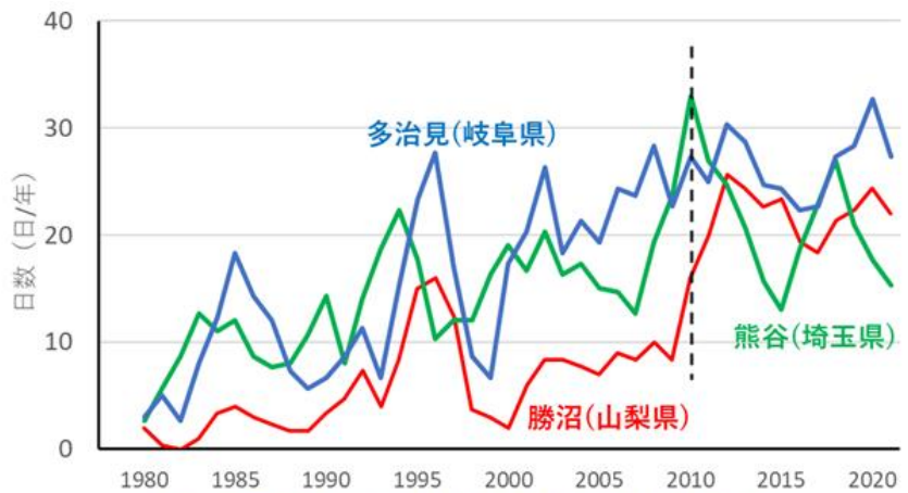
図. 最高気温が35℃以上の日数 (3年移動平均)
